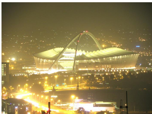
Fot. 8. Stadion zbudowany na XIX Mistrzostwa Świata w Piłce Nożnej w 2010 r. Przezroczysty dach stadionu z teflonu i włókna szklanego ma powierzchnię 46 tys. m 2 . Durban .
